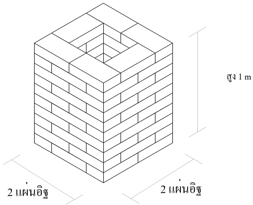
ขยายแสดงการก่อเสาสี่เหลี่ยม 6 แผ่นอิฐ
