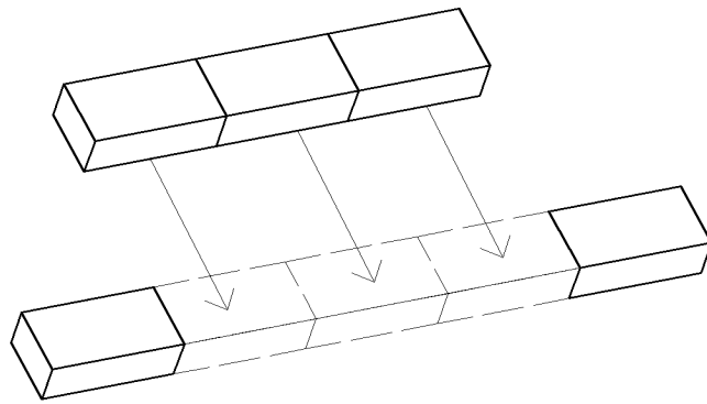
แสดงการก่ออิฐแถวที่ 1,
