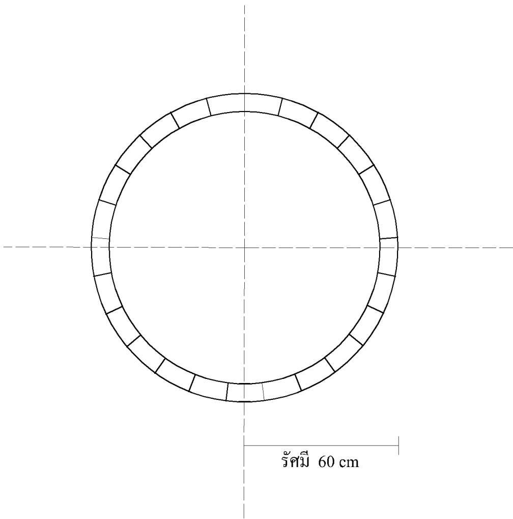
แปลนก่ออิฐวงกลม
