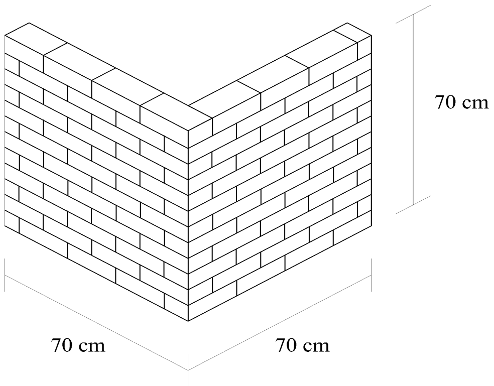
แสดงการก่ออิฐเข้ามุม
