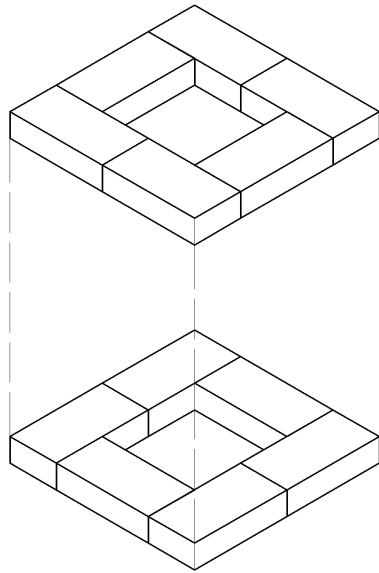
ขยายแสดงการวางอิฐ
