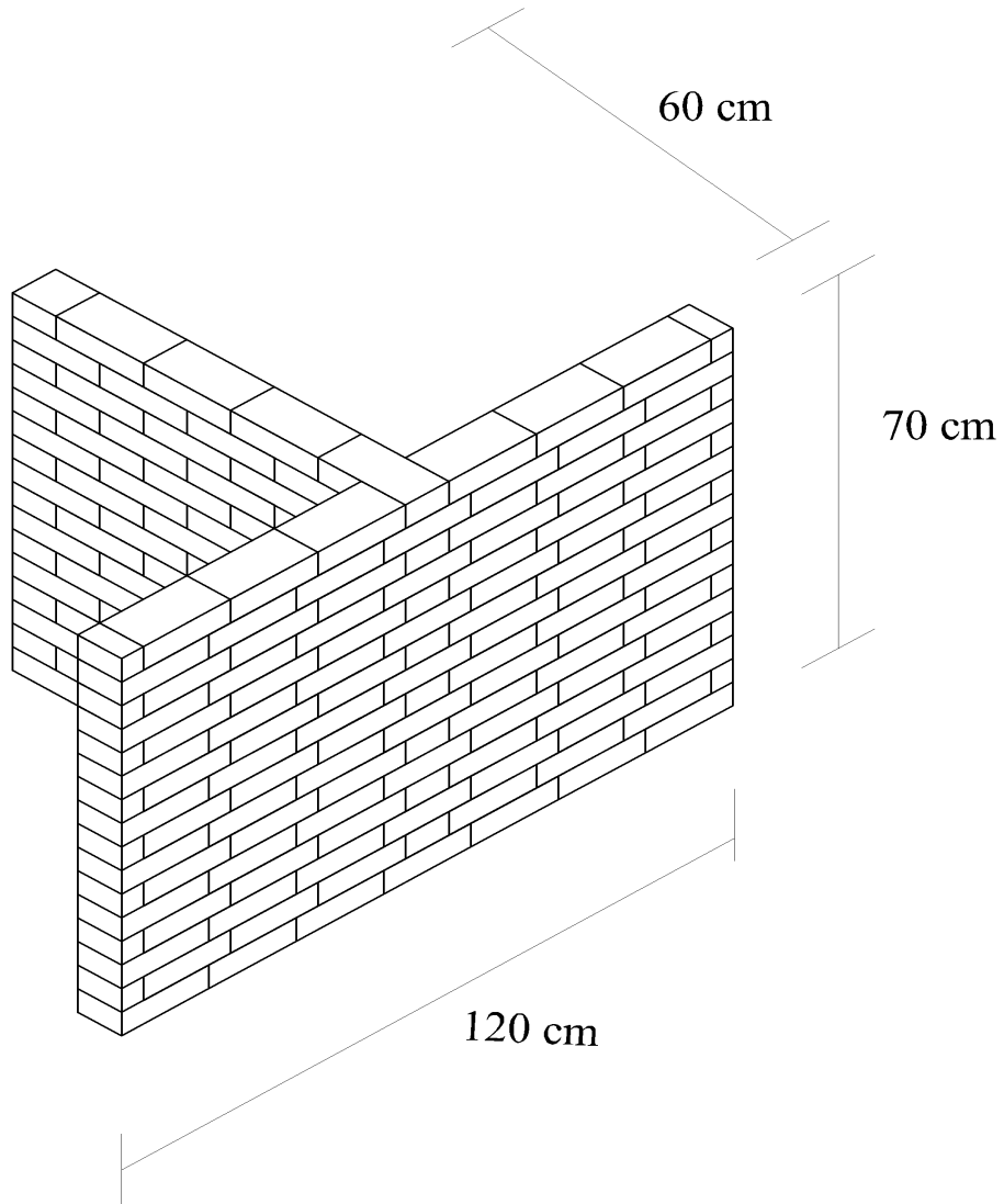
ขยายแสดงการก่อแยกในผนังครึ่งแผ่นอิฐ
