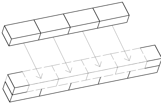
แสดงการก่ออิฐแถวที่ 2,
