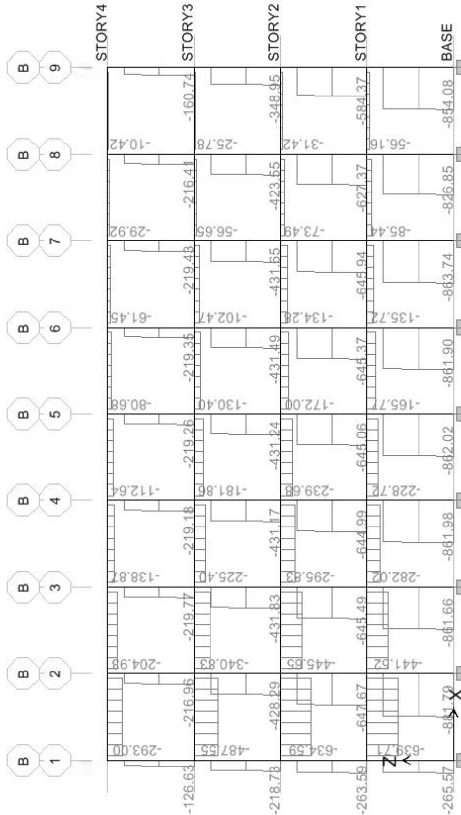
รูปที่ ข.1-7 กระจายแรงแรงในแนวแกนสำหรับโครงในแกน B (กิโลนิวตัน)
