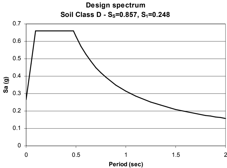
รูปที่ ข.2-1 ตัวอย่างความเร่งตอบสนองเชิงสเปกตรัมเพื่อการออกแบบ สำหรับที่ดั่งบนดินแน่น
