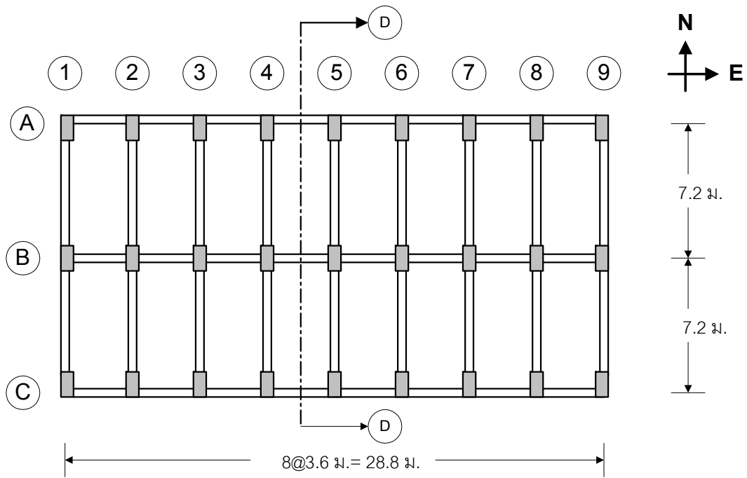
รูปที่ ข.1-1 ผังอาคารของอาคารโรงพยาบาล
