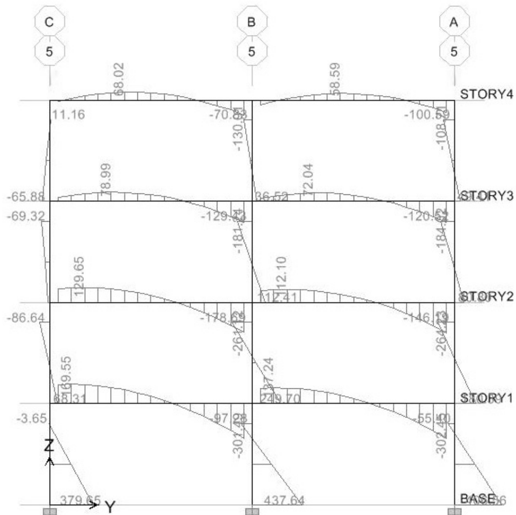
รูปที่ ข.1-5 ไดอะแกรมของโมเมนต์ดัดสำหรับโครงในแกน 5 (กิโลนิวตัน-ม.)
