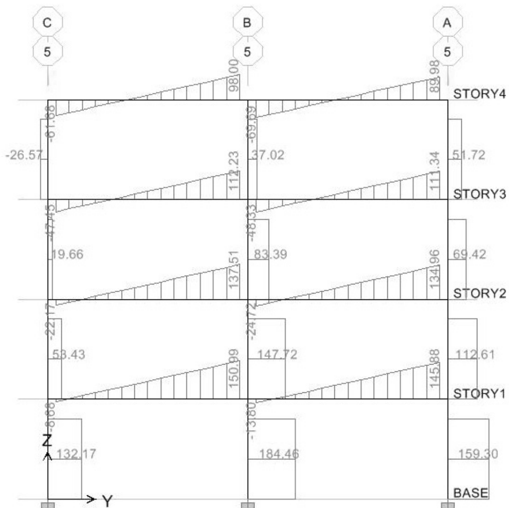
รูปที่ ข.1-6 ไดอะแกรมของแรงเค้นสำหรับโครงในแกน 5 (กิโลนิวตัน)
