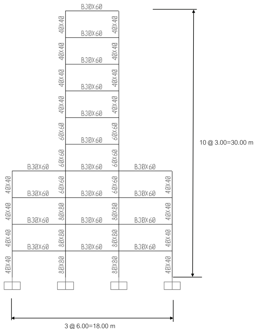
รูปที่ ข.2-3 โครงด้านแรงคัต 2 มิติ ซึ่งมีความไม่สม่ำเสมอในแนวดิ่ง มีขนาดหน้าตัดดังแสดงในรูป
