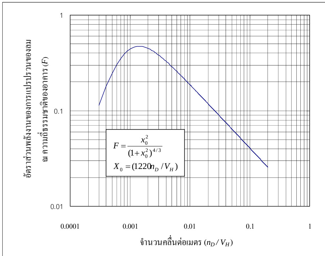
รูปที่ 3.3 แผนภูมิเพื่อหาค่าอัตราส่วนพลังงานของการแปรปรวนของลม ณ ความถี่ธรรมชาติของอาคาร ( F ) ซึ่งเป็นฟังก์ชันของจำนวนคลื่นต่อเมตร
