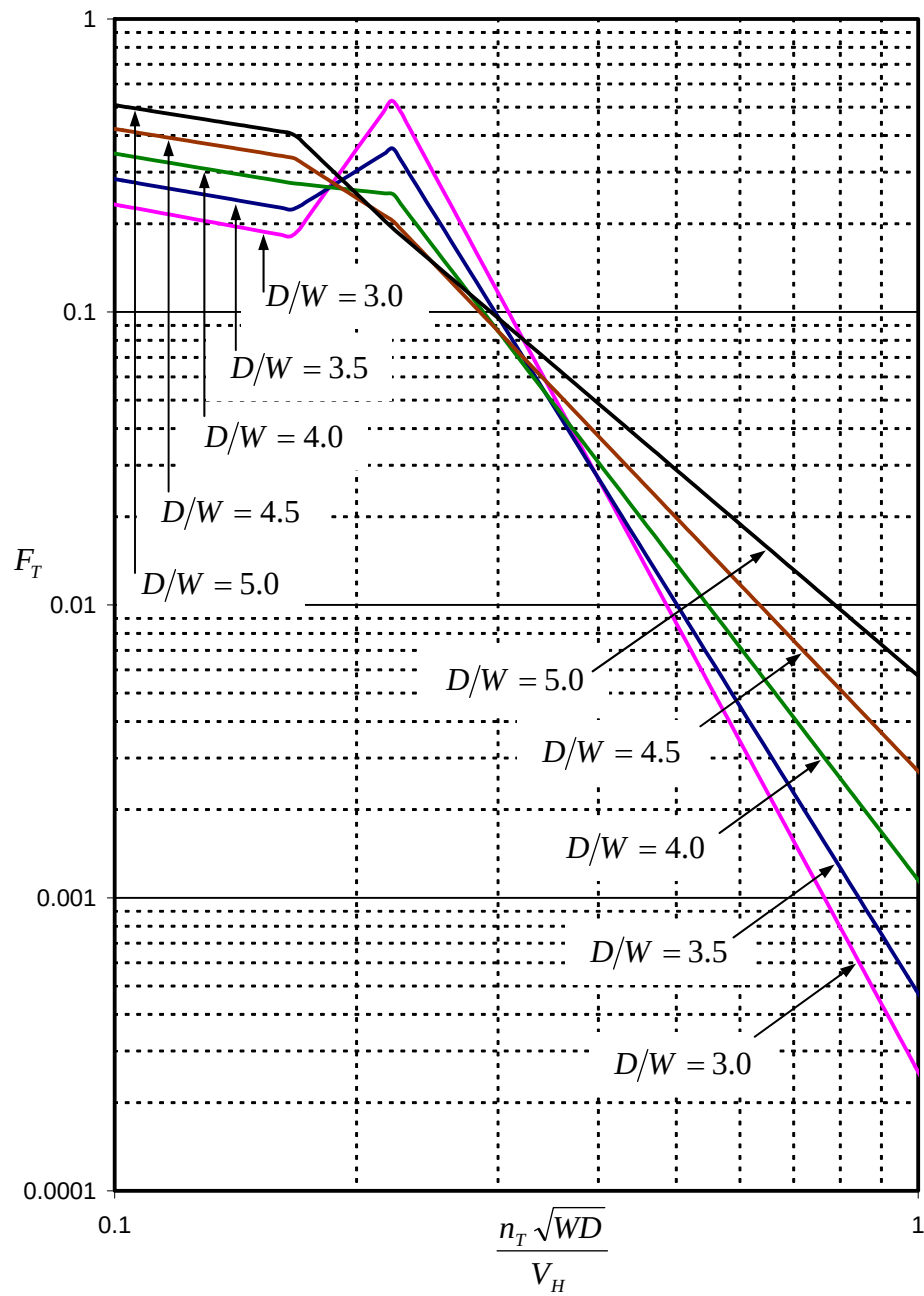
รูปที่ 4.8 สเปกตรัมของแรงลมในแนวนิของอาคาร สำหรับ D/W = 3.0, 3.5, 4.0, 4.5 และ 5.0
